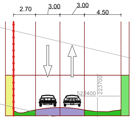
SECTIUNE A-A
